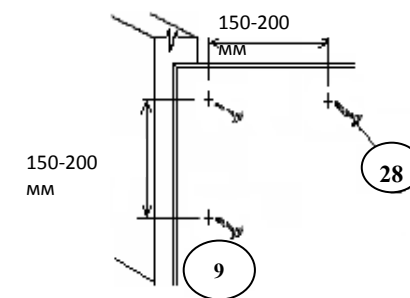
Рис. 2 Крепление дна ящика
